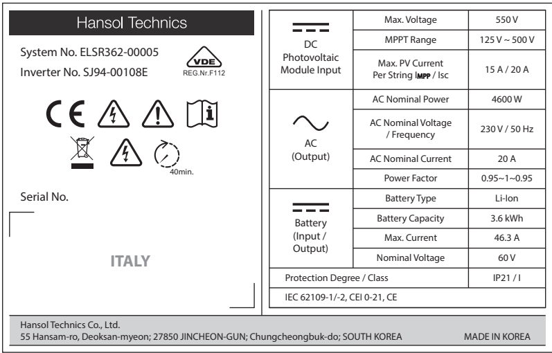
[Figura 2-2: Targhetta di identificazione]
