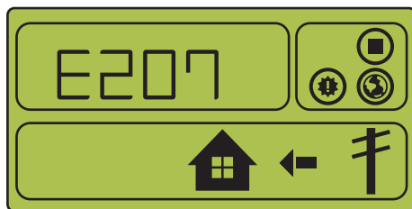
[Figura 4-24: Occorrenza di evento, evento di collegamento CC inverter normale]
