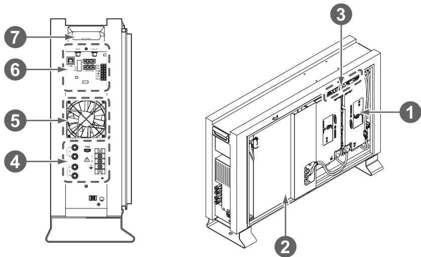
[Figura 3-1: Vista delle parti di Q.HOME+ ESS-G1 5.5]
