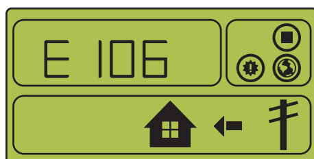
[Figura 4-17: Occorrenza di evento, protezione per sovracorrente stringa PV 1]
