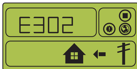
[Figura 4-26: Occorrenza di evento, evento di collegamento CC inverter in sequenza]
