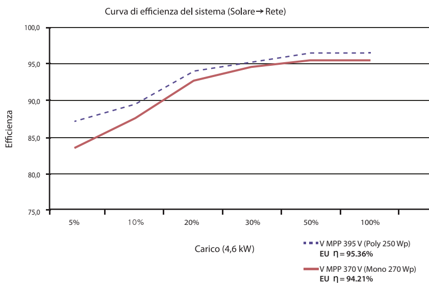
[Figura 2-7: Curva di efficienza della potenza della generazione e PV]
