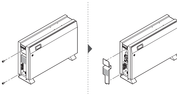
[Figura 6-1: Rimozione del pannello laterale]
