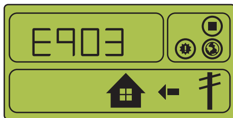
[Figura 4-33: Occorrenza di evento, evento di guasto singolo]
