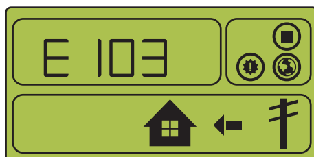
[Figura 4-14: Occorrenza di evento, protezione per collegamento inverso stringa PV 1]
