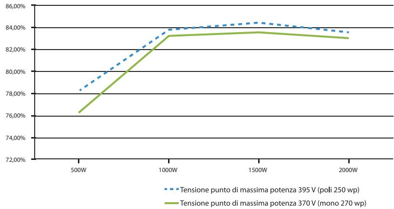
[Figura 2-6: Curva di efficienza della potenza del sistema]
