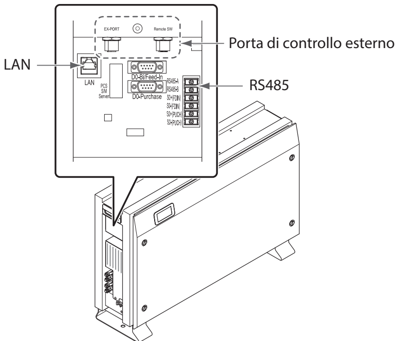
[Figura 5-1: Morsetto di comunicazione]
